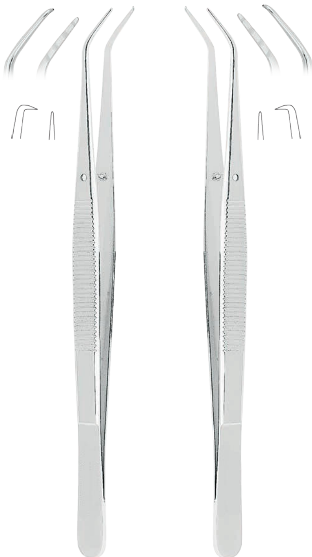
2512 Fig. 1 Goldman-Fox cm.15
